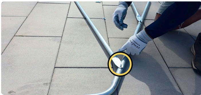
Fixation du rail de porte au coin EA / Door rail fastened to the corner EA
