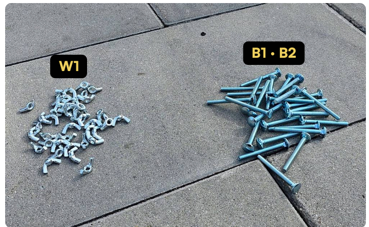
Papillons W1 • boulons B1 B2 / Wing nuts W1 • bolts B1 B2
